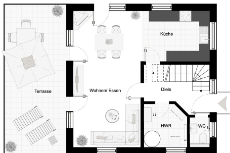
Grundriss Erdgeschoss
