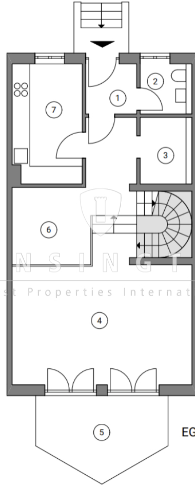
Grundriss EG
