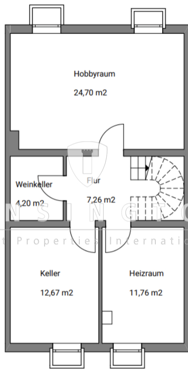
KG
